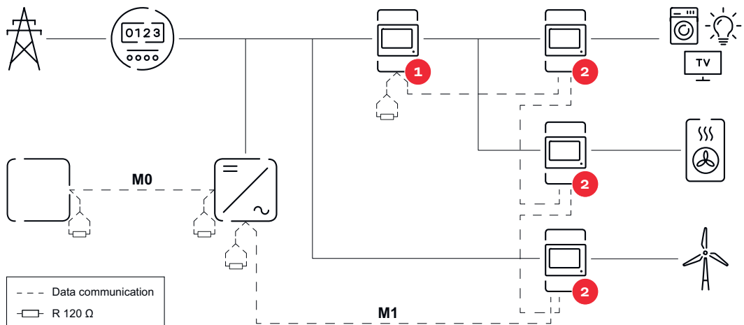
Position des Primärzählers im Verbrauchsweig. *Abschluss-Widerstand R 120 Ohm
